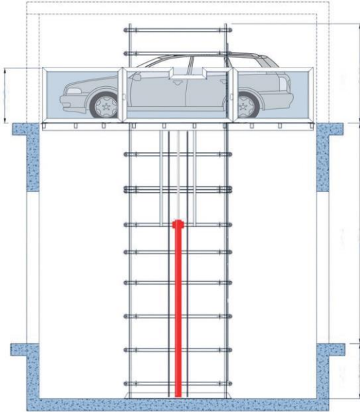
Sektionsansicht – HOCH
