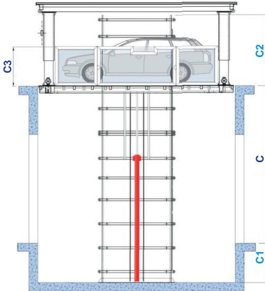
Sektionsansicht – HOCH
