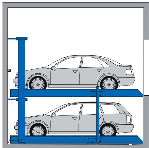
maszyna w pozycji opuszczonej
