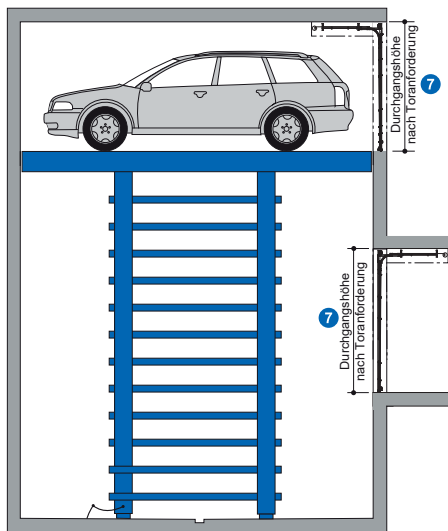
Garagen-Sektionaltor
